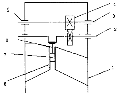
1、机身 2、曲轴 3、输入轴 4、齿轮副 5、轴承 6、连杆 7、滑块 8、导轨
